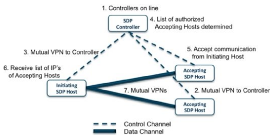
[그림 1] SDP Workflow
